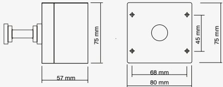
简易仪器 GRP 接线盒，带尼龙接地夹存储销
