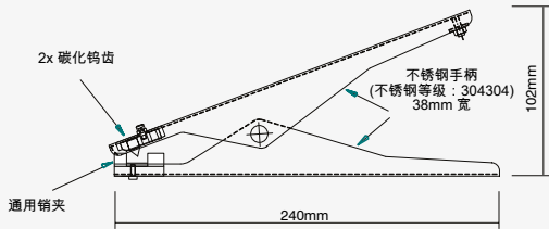
配备一对碳化钨尖的双芯不锈钢接地夹
